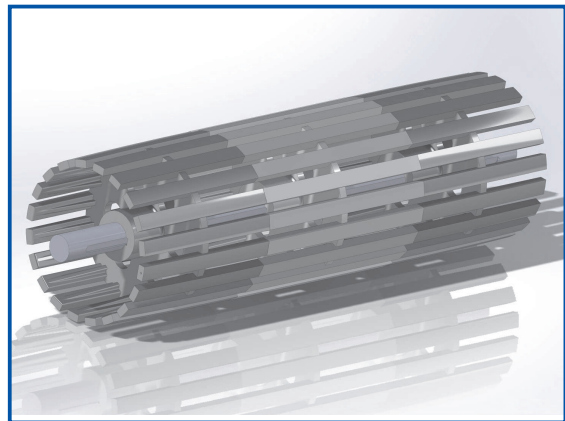
Kombination von drei Stabtrommeln für Förderanlage
